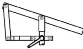
Låsbar spak
